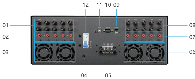
01 Output输出端子 (CH1-CH5) 02 SENSE补偿接口 (宽范围机型支持选配) 03 风扇散热口 04 接地端子 05 电源输入接口 06 风扇散热口 07 SENSE补偿接口 (宽范围机型支持选配) 08 Output输出端子 (CH6-CH10) 09 RS485通信接口 10 RS232通信接口 11 USB通信接口 12 断路器
